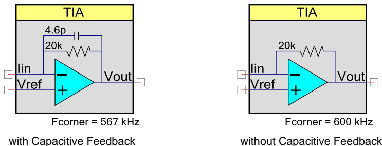
图 1. TIA 配置
