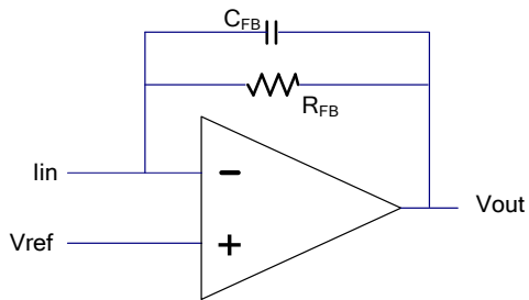
图 2. TIA 原理图
