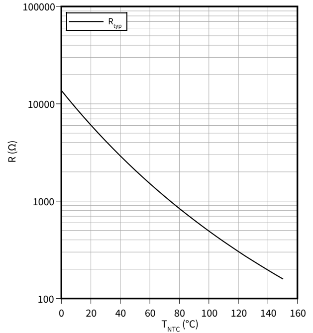
サーミスタの温度特性, NTC-サーミスタ
