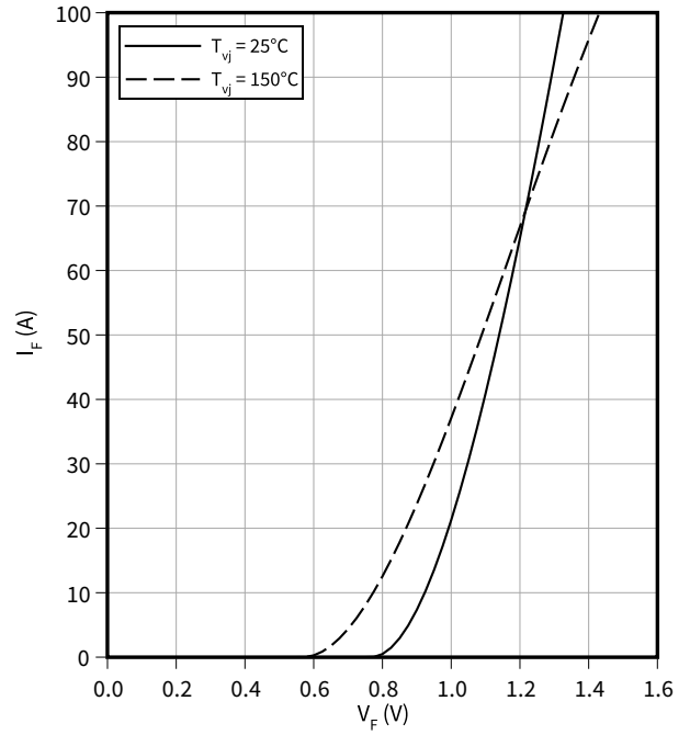
正向特性 (典型), 二极管, 制动-斩波器
